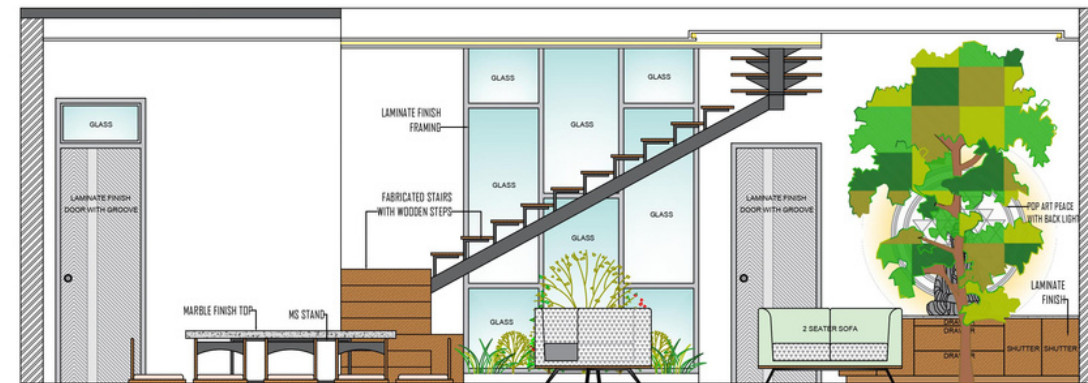
ELEVATION-A
